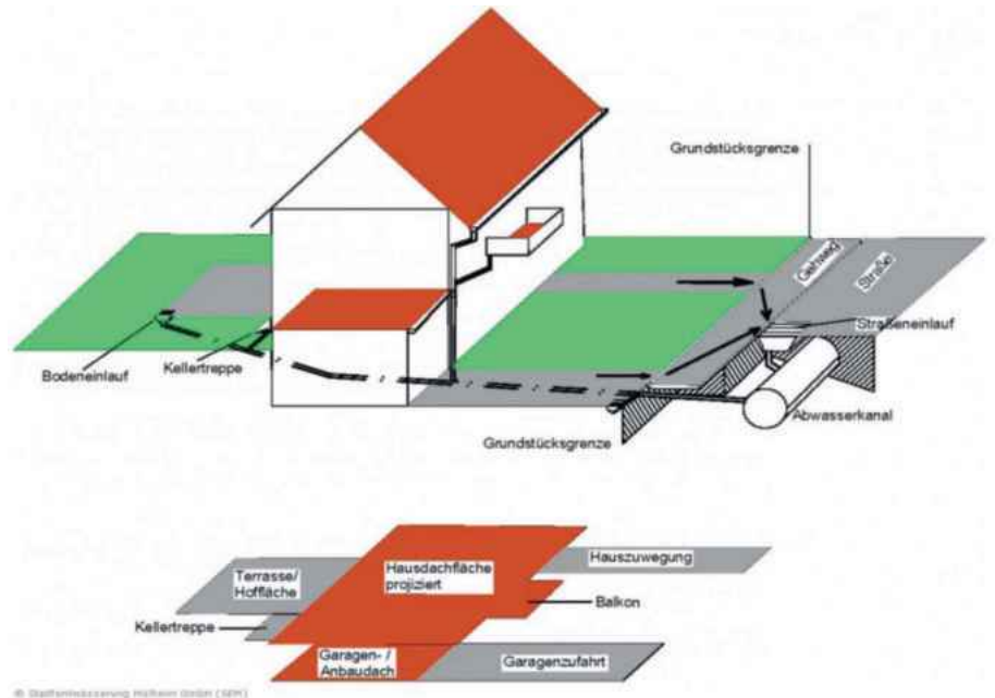
An die Grundstücksentwässerung angeschlossene und nicht angeschlossene Flächen
